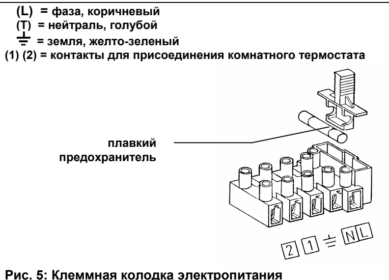
Рис. 5: Клеммная колодка электропитания
