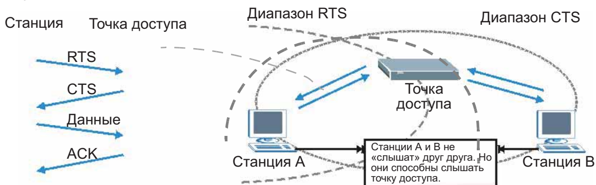
Рисунок 235 RTS/CTS
