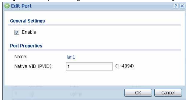
Рисунок 50 Экран Configuration > Wireless > AP Management > Edit AP List > Edit Port
