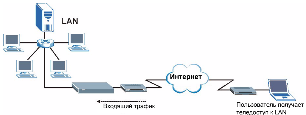
Рис. 61 Настройка Telnet в сети TCP/IP
