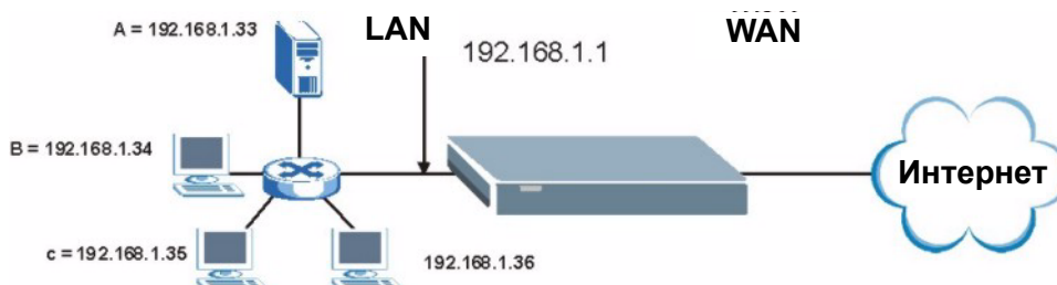
Рис. 39 Пример: Несколько серверов расположены за NAT
