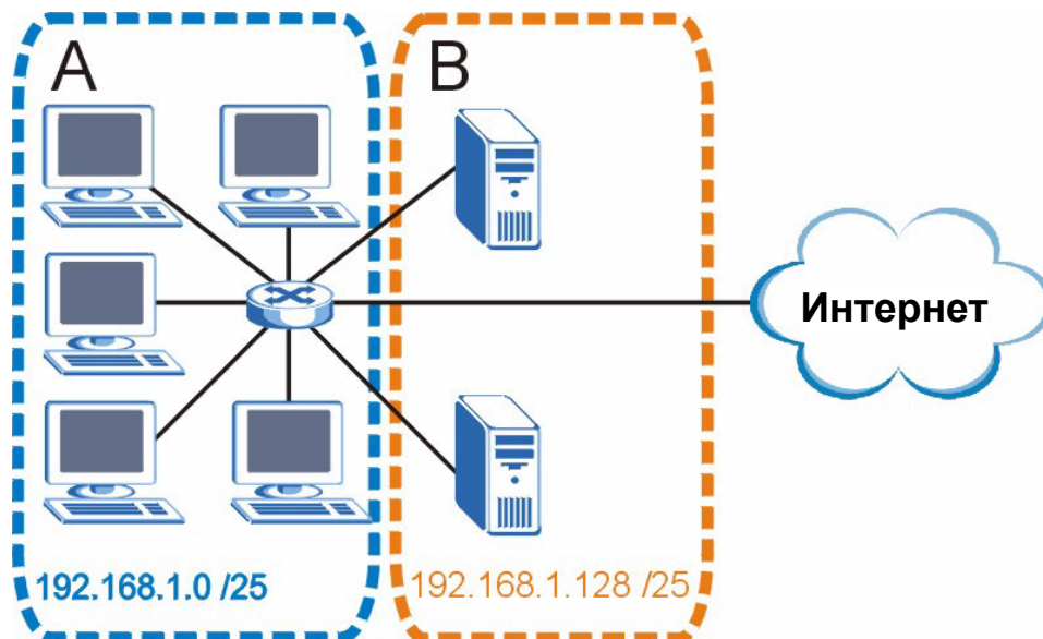
Рис. 105 Пример организации подсетей: после разделения на подсети
