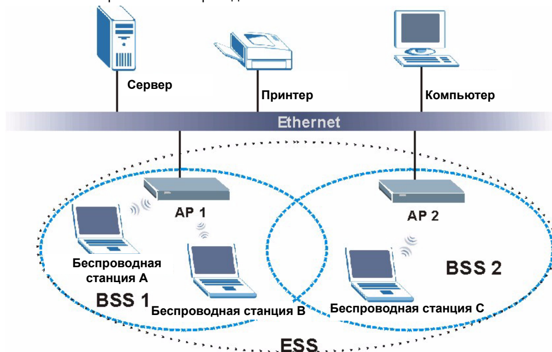
Рис. 131 Фиксированная беспроводная сеть
