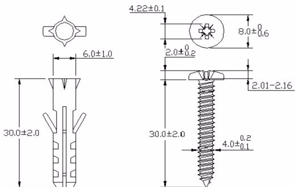
Рис. 94 Дюбель и винт с резьбой М4
