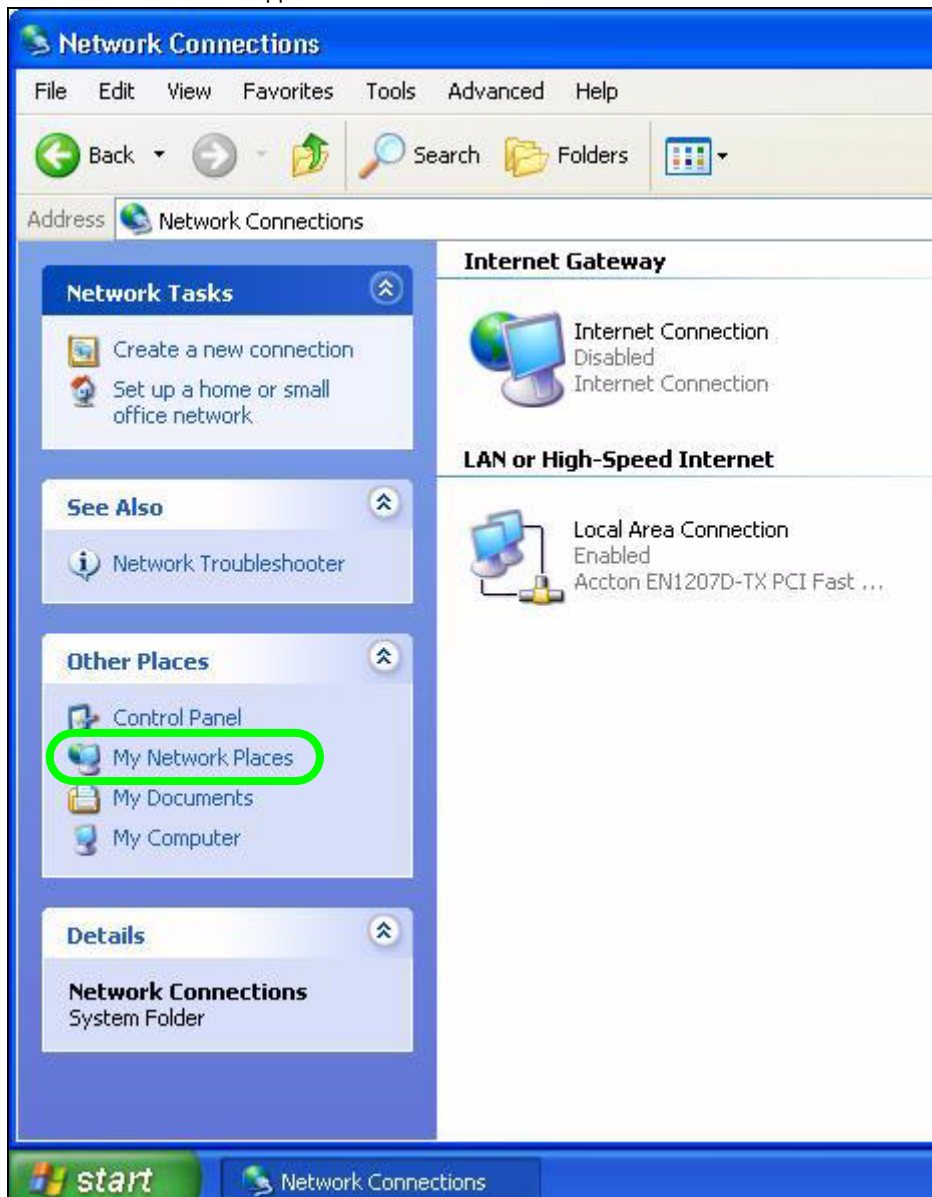
Рис. 77 Сетевые подключения
