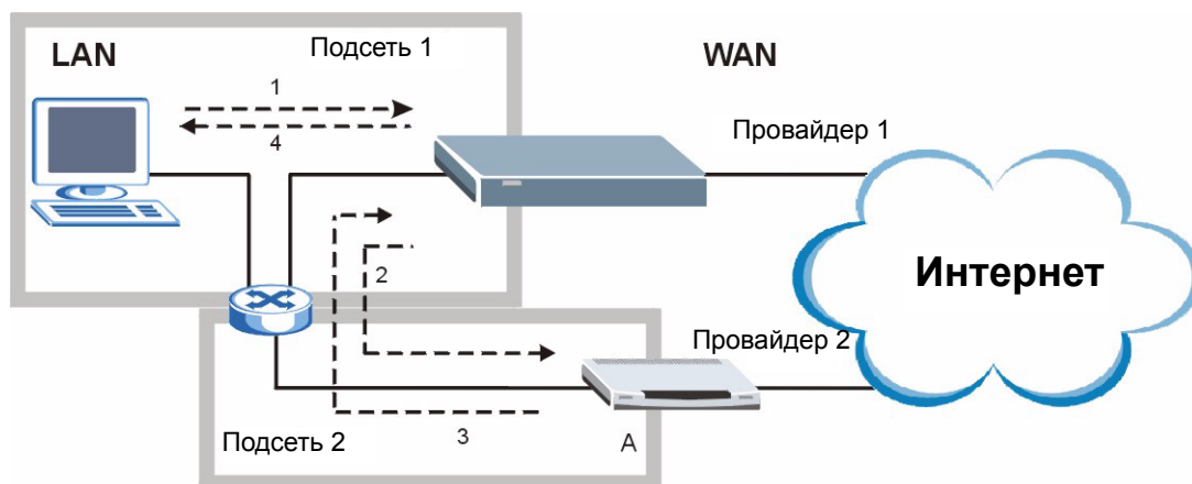
Рис. 46 Использование псевдонима IP для решения проблемы треугольного маршрута
