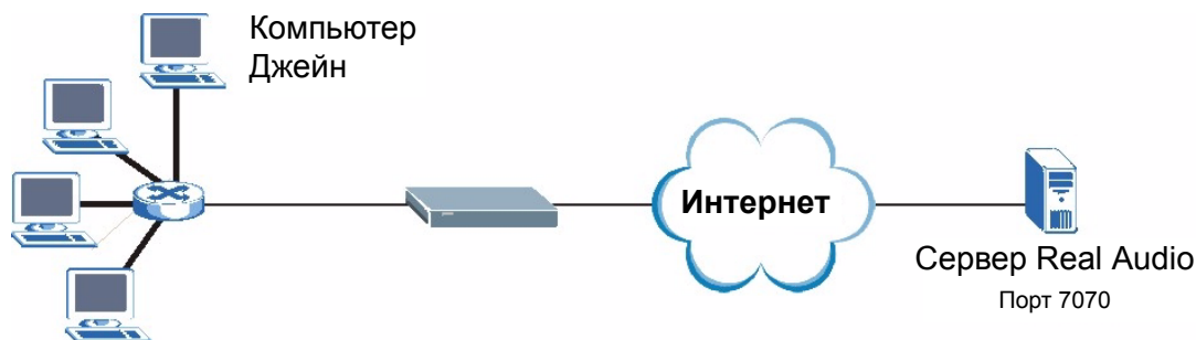
Рис. 43 Пример процесса инициации переадресации портов
