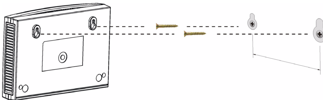
Рис. 93 Пример настенного монтажа
