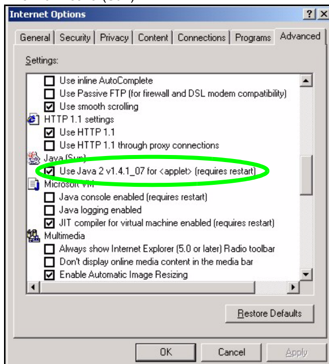
Рис. 102 Java (Sun)
