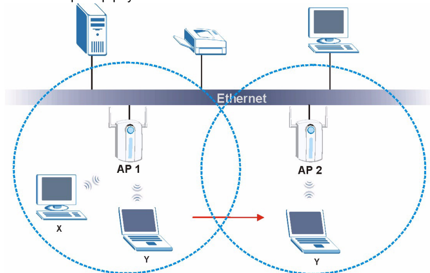
Рис. 18 Пример роуминга
