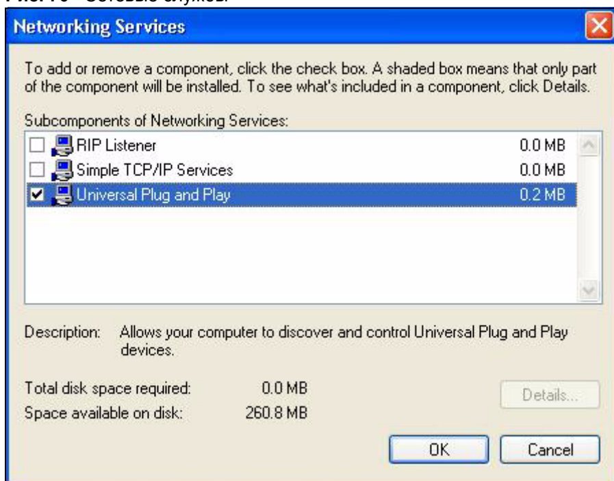
Рис. 70 Сетевые службы
