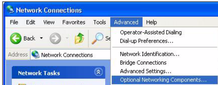
Рис. 68 Сетевые подключения
