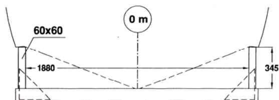
Размеры киль-блоков для судна Yamarin 64 Day Cruiser
