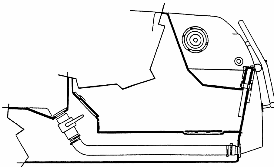
Расположение кингстонов и клапанов судна Yamarin 44 Side Console
