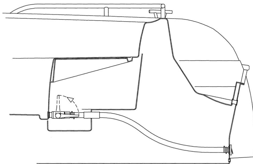
Расположение кингстонов и клапанов судна Yamarin 46 Side Console
