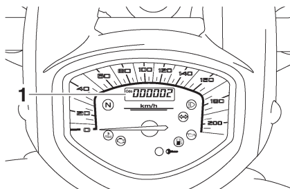
1. Одометр/счетчик пути за поездку/счетчик пути на остатке топлива/часы
