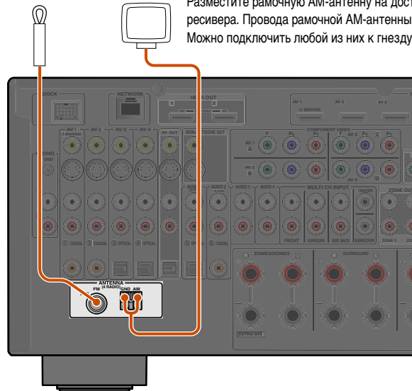
Рамочная AM-антенна
