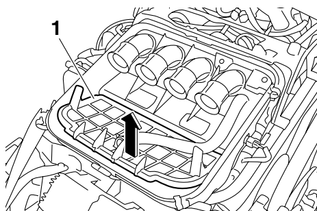
1. Рама фильтрующего элемента
