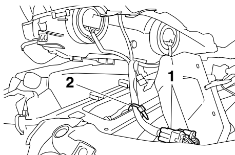
1. Электрический разъем фар 2. Пластмассовый поясок
