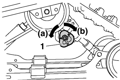
1. Регулятор предварительного натяжения пружин
