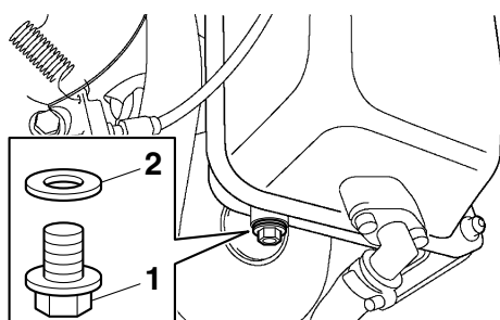
1. Болт слива моторного масла (из масляного бака) 2. Прокладка
