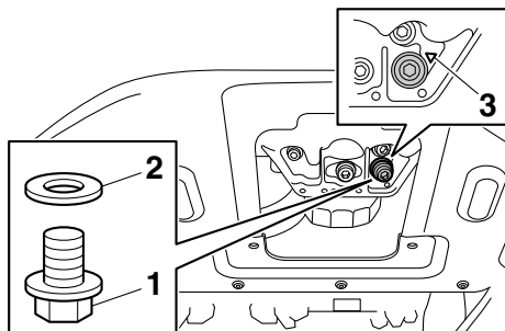
1. Болт слива моторного масла (из картера) 2. Прокладка 3. Отметка “▽”
