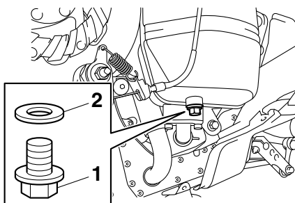
1. Болт слива моторного масла (из масляного бака) 2. Прокладка
