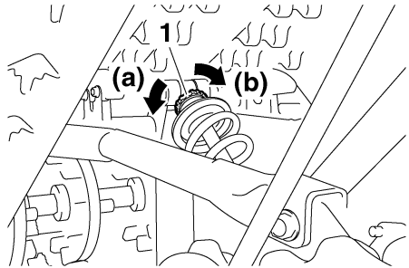
1. Лимб регулировки демпфирующей силы отбоя
