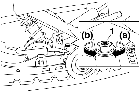
1. Регулировочный винт демпфирующей силы сжатия
