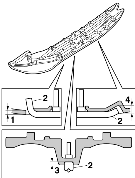
1. Предел износа полозьев
