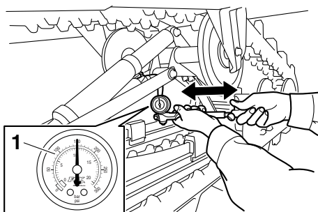
1. Манометр (шкала высокого давления)
