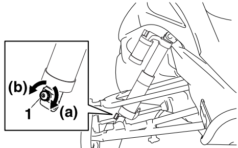
1. Ручка регулировки демпфирующей силы отбоя
