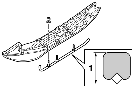
1. Предел износа полозьев
