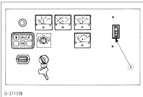
(1) 断路器开关
