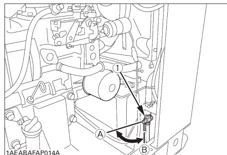
(1) Robinet de vidange d'eau
