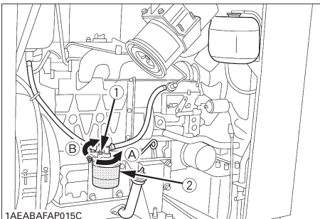
1AEABAFAP015C (1) Tapón de purga de aire (A) "ABRA" (2) Cartucho del filtro de combustible (B) "CIERRE"
