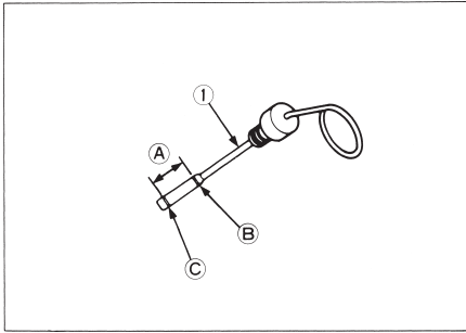
(1) مقياس عمق الزيت (A) "مستوى الزيت المناسب" (B) "المستوى العلوي" (C) "المستوى المنخفض"
