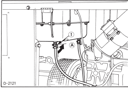
(1) صنوبر خزان الوقود (A) "غلق"
