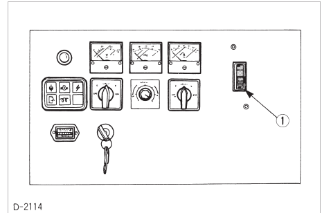
(1) Coupe-circuit
