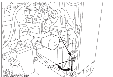
1AEABAFAP014A (1) Grifo de drenaje de agua (A) "ABIERTO" (B) "CERRADO"
