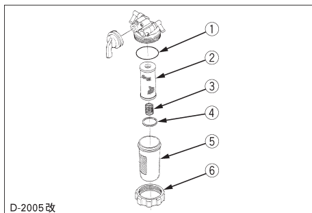
D-2005改 (1) Junta tórica (2) Elemento del filtro (3) Muelle (4) Taza del filtro (5) Aro roscado (6) Marcador
