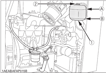
1AEABAFAP015B (1) Расширительный бачок (А) «FULL» верхняя линия 1,1 л (2) Крышка (В) «LOW» (низкий уровень)
