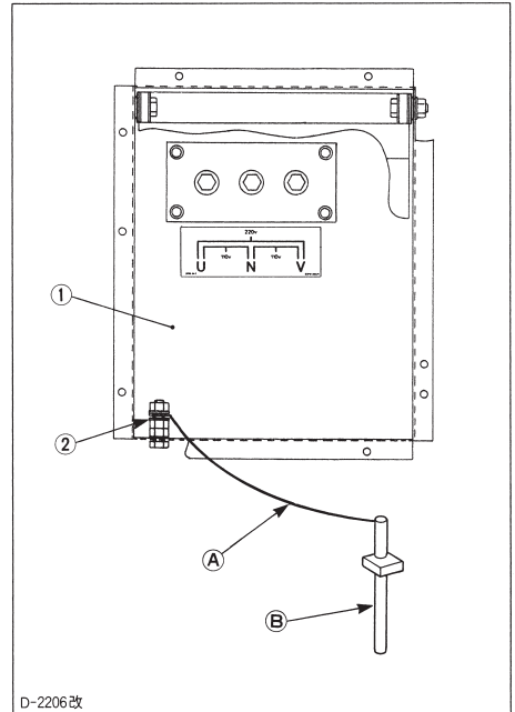
D-2206改 (1) Tapa centro de carga (A) #6AWG Conexión a tierra de cobre flexible (2) Terminal de conexión a tierra del generador (B) Varilla de conexión a tierra de metal o sistema de la tubería de agua corriente del edificio, de acuerdo a los códigos de N.E.C.
