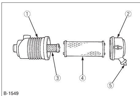
B-1549 (1) 空气滤清器机体 (2) 盖 (3) 二级滤芯 (4) 主滤芯 (5) 排空阀
