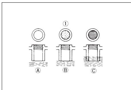
(1) 电解液液面
