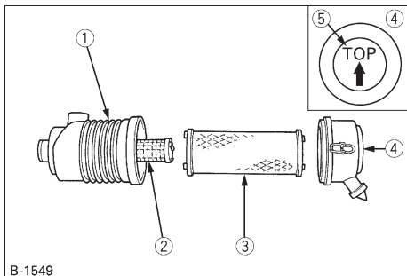
B-1549 (1) 空气滤清器机体 (2) 二级滤芯 (3) 主滤芯 (4) 集尘碗 (5) “TOP”（上方位）标记
