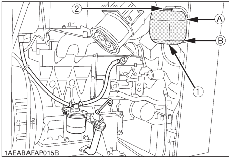
1AEABAFAP015B (1) Réservoir de réserve (A) « FULL » (2) Bouchon Repère supérieur 1,1 l (B) « LOW »
