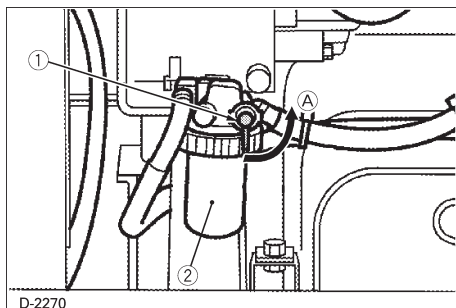
(1) Palanca de combustible (A) "CLOSE" (2) Separador de agua
