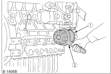
(1) خزانة فلتر الزيت (2) انزع باستخدام مفتاح ربط المشح (اربطه بيدك بالحكم)
