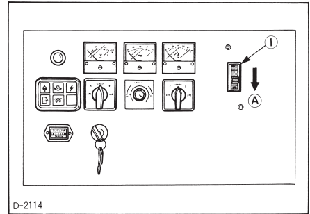
(1) قاطع الدائرة الرئيسي (A) "إيقاف"
