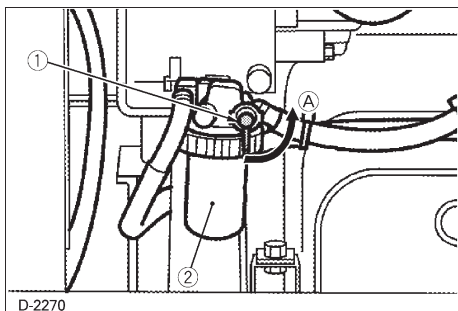
D-2270 (1) 燃油箱旋阀 (A) “关闭” (2) 油水分离器
