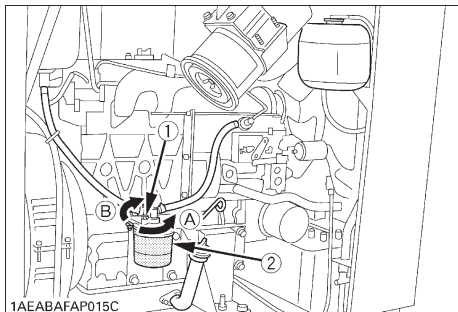
(1) 排气塞
