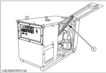
(1) Упор дверцы
