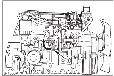
B-1555A (1) Palanca de parada (A) "PARADA"
