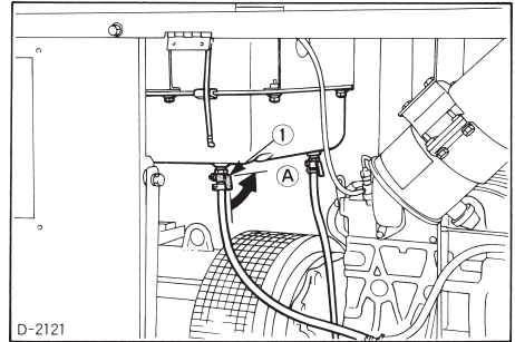
(1) Кран топливного бака (A) «CLOSE» (закр.)
