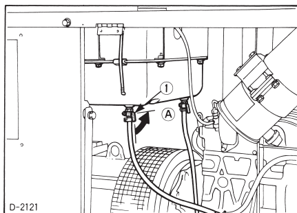
(1) Grifo del depósito de combustible
