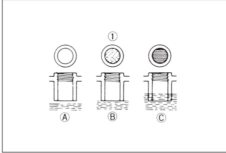
(1) مستوى سائل البطارية (A) "منخفض جدا" (B) "مناسب" (C) "مرتفع جدا"
