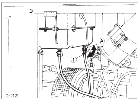
(1) 燃油箱栓
