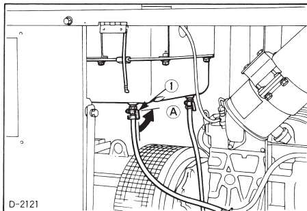
(1) Robinet d'alimentation
