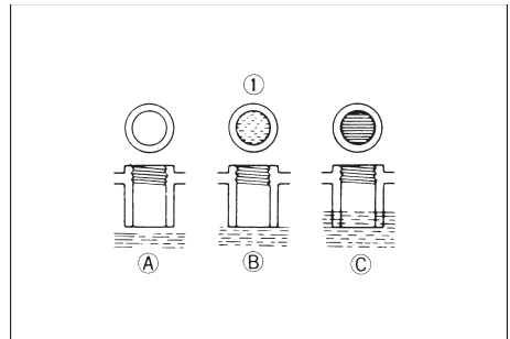
(1) Уровень электролита в аккумуляторе (А) «СЛИШКОМ НИЗКИЙ» (В) «ПРАВИЛЬНЫЙ» (С) «СЛИШКОМ ВЫСОКИЙ»
