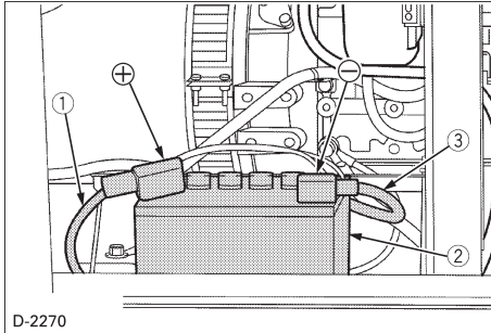
(1) الكيل السميكة الأحمر + (2) صندوق البطارية (3) الكيل الأسود السالب/الأرضي -
