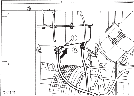
D-2121 (1) Grifo del depósito de combustible (A) "CIERRE"
