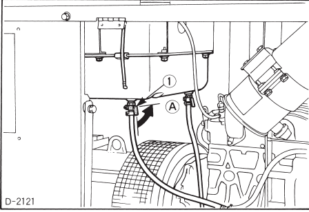
(1) صنبور خزان الوقود (A) "إغلاق"
