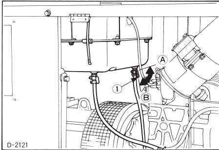
(1) صنبور تصريف خزان الوقود (A) "إفتح" (B) "أغلق"
