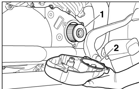
1. Фильтрующий элемент масляного фильтра 2. Уплотнительное кольцо
