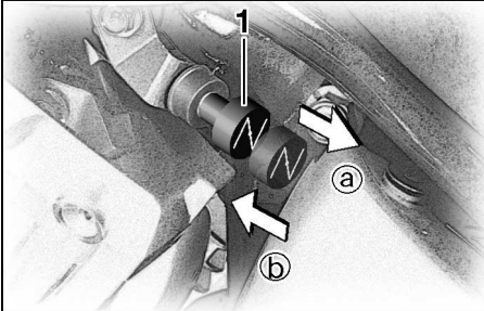
1. Ручка пускового устройства (воздушной заслонки) "1\1"
