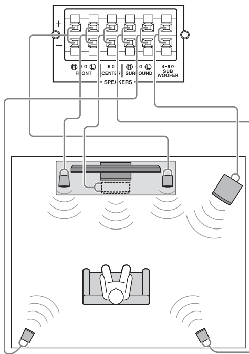
本机后面板 (当超低音扬声器为无源时)
