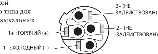
Разъем Neutrik NL4FC
