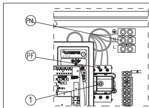
Подключение котла к трехфазной электросети.
