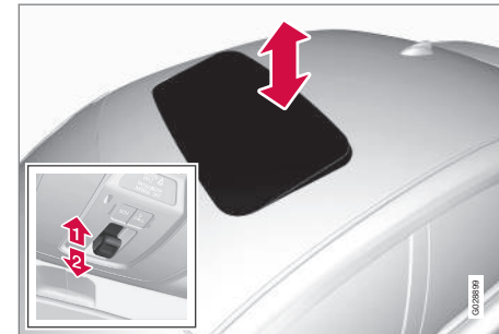
Вертикальное открытие, задний край вверх.
