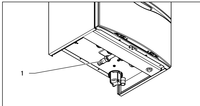
Рис. 5.1 Подсоединение газа (пример: аппарат VUV)
