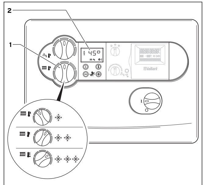
Εικ. 4.8 Ρύθμιση της θερμοκρασίας εξόδου χωρίς ρυθμιστική συσκευή
