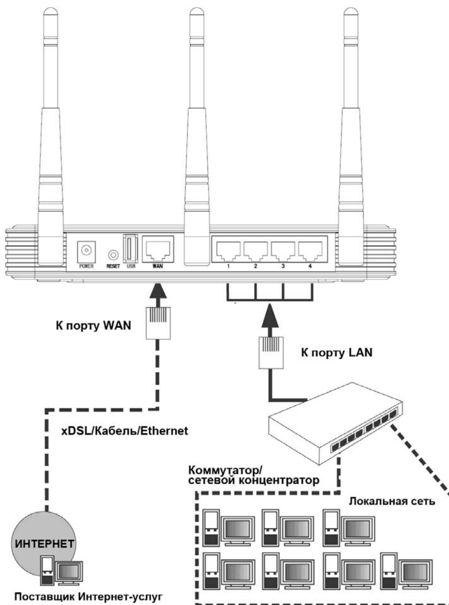
Рис. 2-1 Установка аппаратной части маршрутизатора
