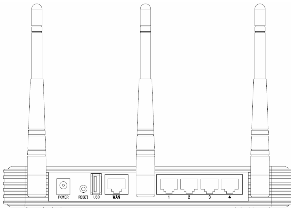
Рис. 1-2 Задняя панель
