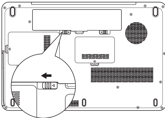
Рисунок 6-1 Высвобождение батарейного источника питания (1)
