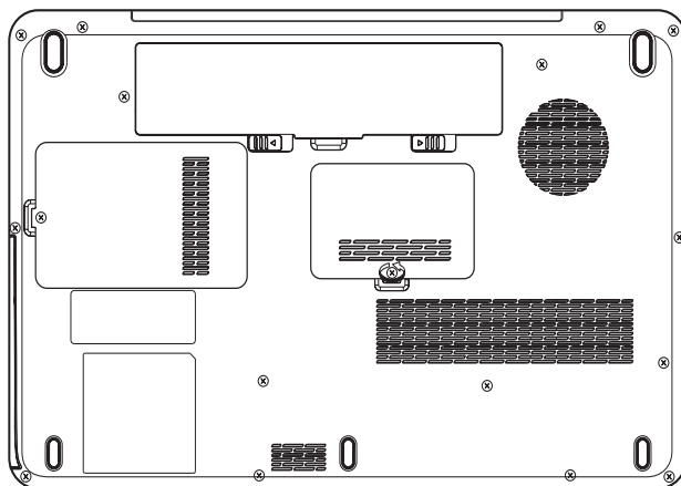
Рисунок 8-3 Устанавливаем крышку отсека для модулей памяти
