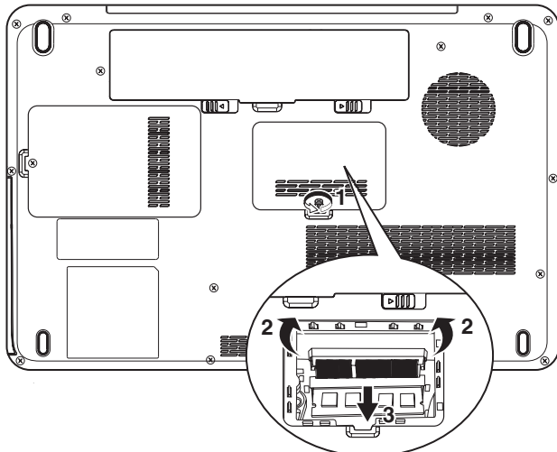
Рисунок 8-2 Снимаем крышку отсека для модулей памяти
