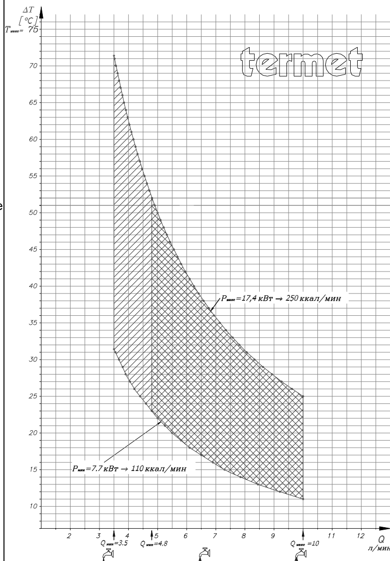
Рис. 4.3.2 Характеристика работы нагревателя
