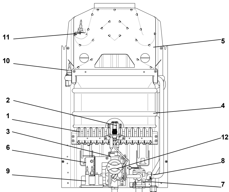
Рис. 2.2.1.1. Главные узлы водонагревателя
