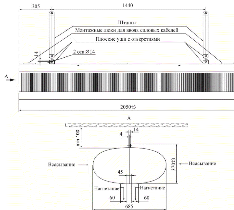
Рис. 7. Крепежные размеры КЭВ-П601Е, КЭВ-П603Е
