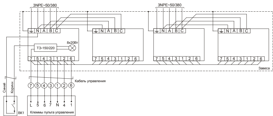
Рис.4. Схема подключения кабеля к пульту управления.
