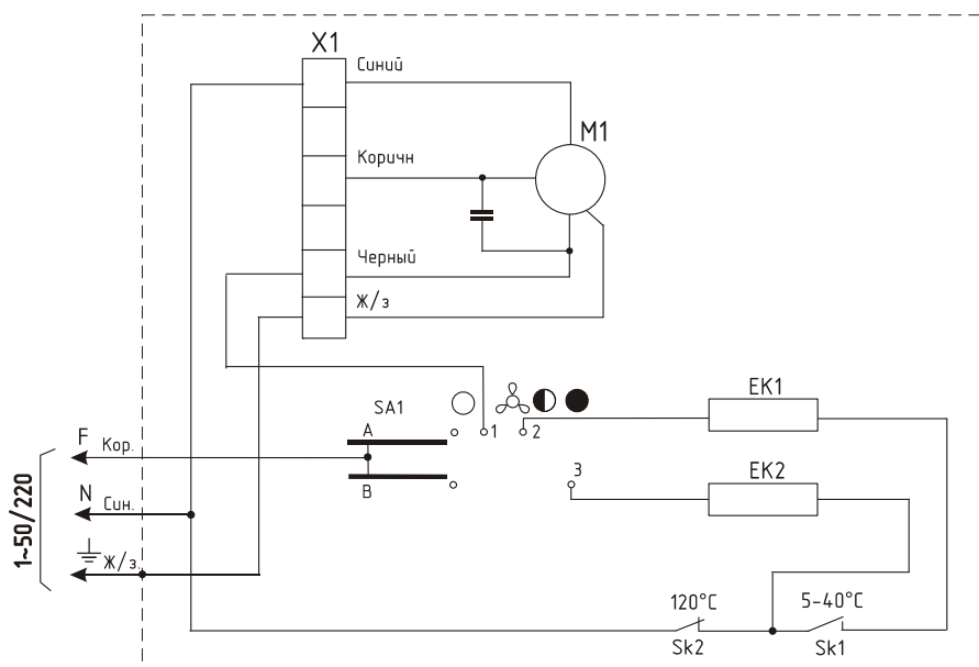
Рис. 7 Электрическая схема завесы КЭВ-4П1150Е
