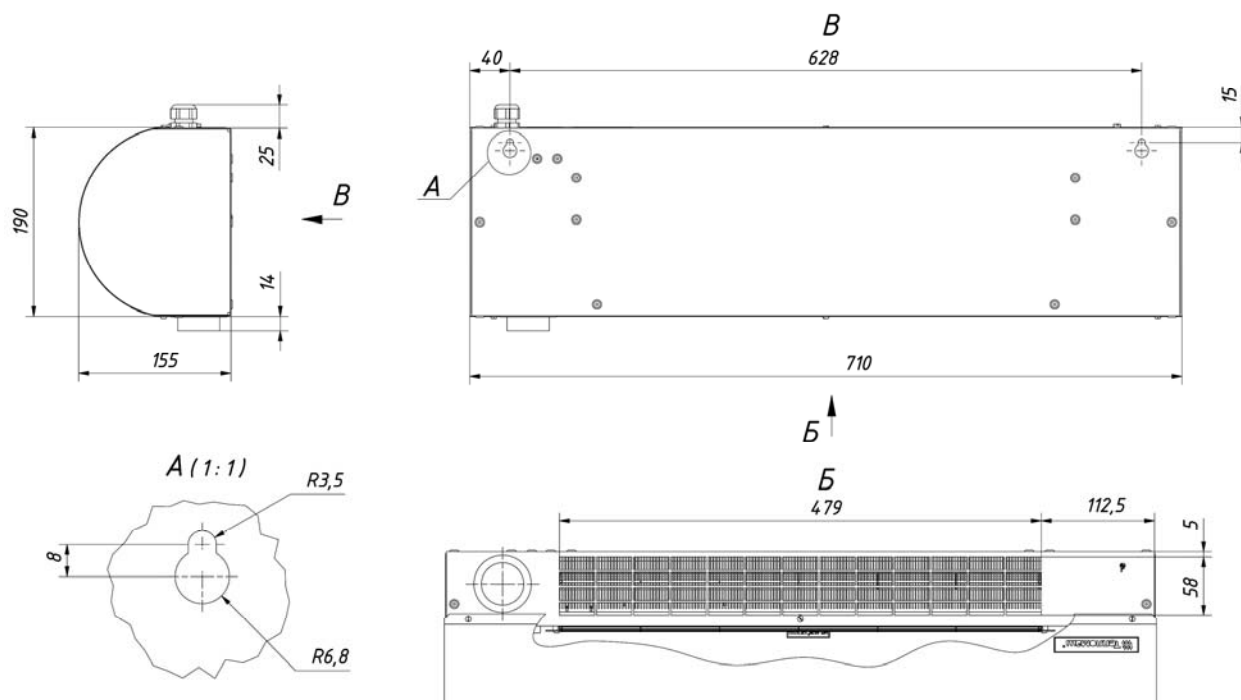
КЭВ-3П1120Е, КЭВ-4П1120Е, КЭВ-5П1120Е
