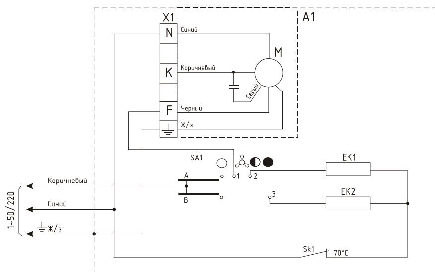
Рис. 2 Электрическая схема занесы КЭВ-3П1120Е
