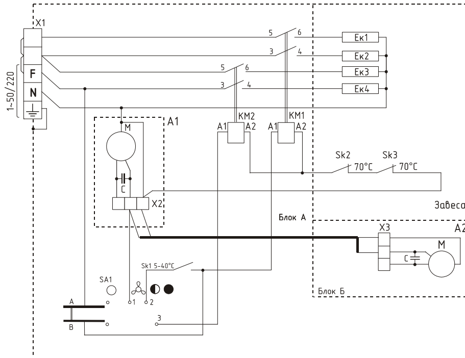
Рис. 10 Электрическая схема завес КЭВ-8П1060Е, КЭВ-10П1060Е
