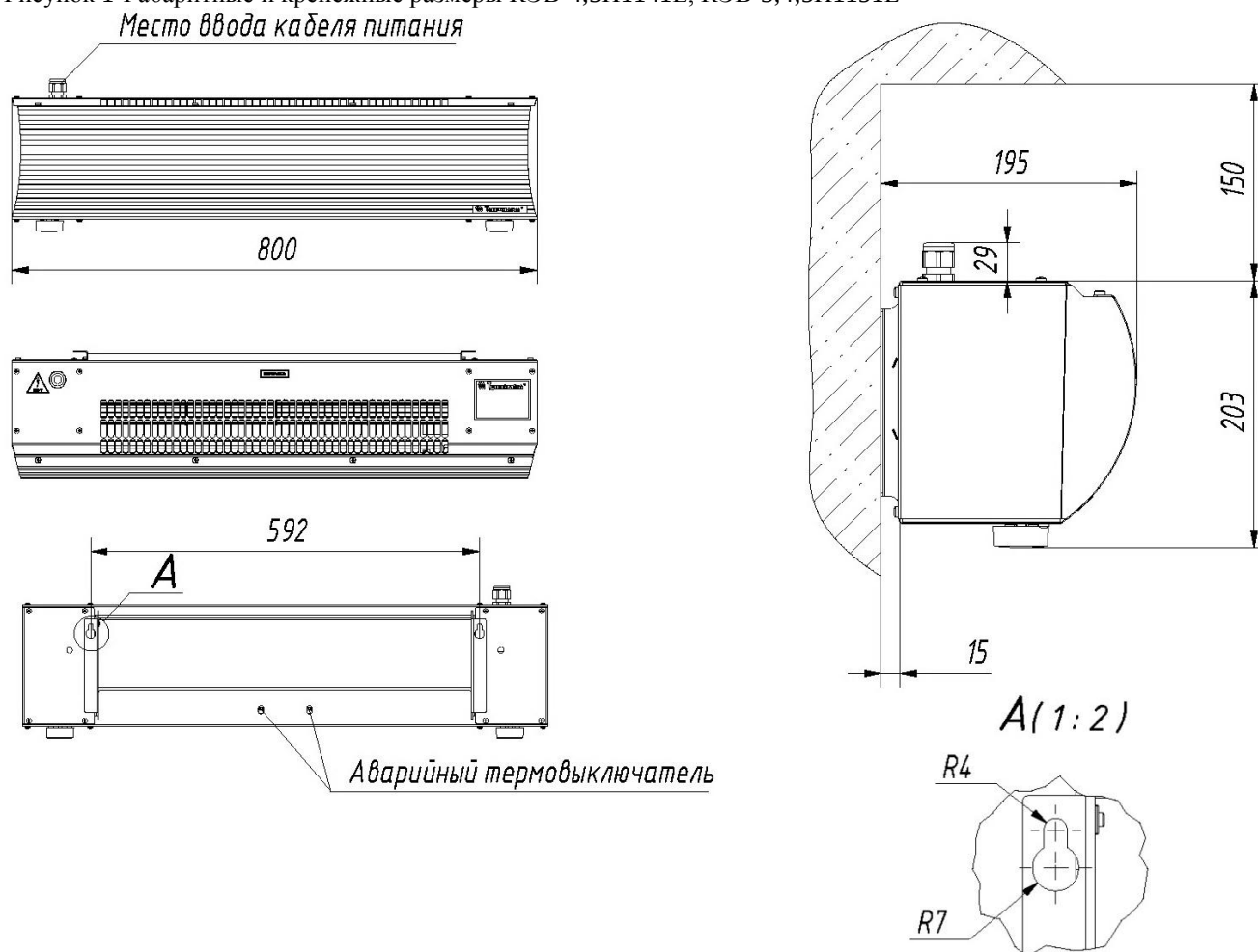
Рисунок 1-Габаритные и крепежные размеры КЭВ-4;5П1141Е, КЭВ-3;4;5П1151Е
