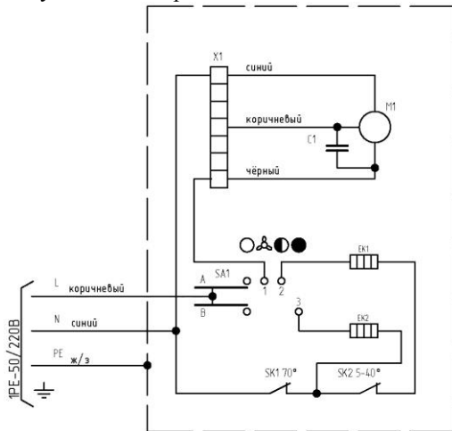
Рисунок 7-Электрическая схема КЭВ-3;4; П1151Е
