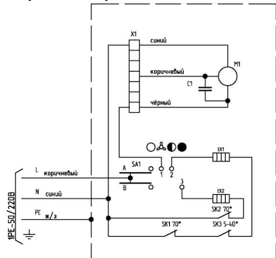
Рисунок 8-Электрическая схема КЭВ-5П1151Е
