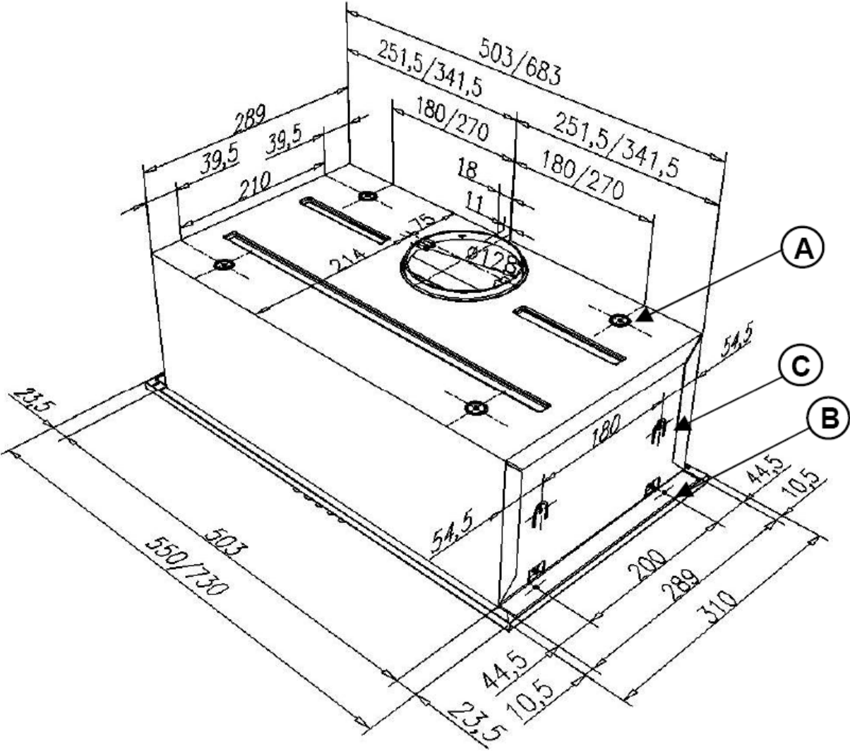
Габариты (мм)
