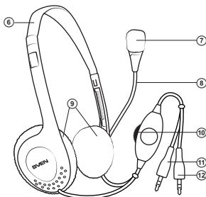
Мал. 2. Стереогарнітура
