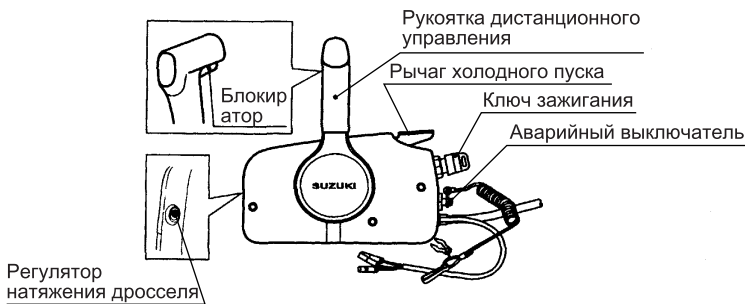
УЗЕЛ ДИСТАНЦИОННОГО УПРАВЛЕНИЯ (DT30R)
