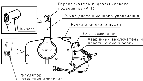
ДИСТАНЦИОННОЕ УПРАВЛЕНИЕ
