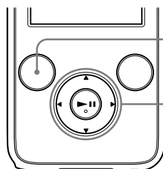
Кнопка BACK/HOME
