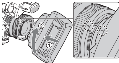
Кнопка PUSH (снятие бленды объектива)
