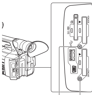
Кнопка гнезда карты памяти A
