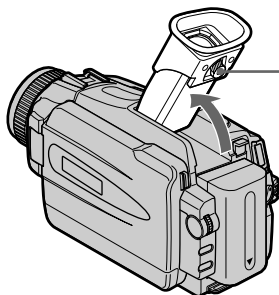
The viewfinder lens adjustment lever/ Рычаг регулировки объектива видоискателя
