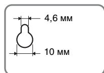
Отверстие в задней панели динамика
