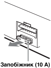
Запобіжник (10 А)
