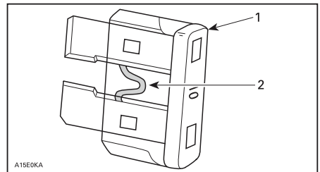
1. Предохранитель
