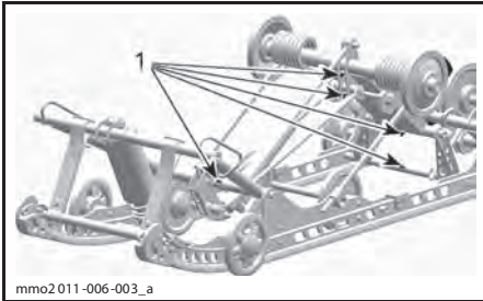
1. Пресс-маслёнки
