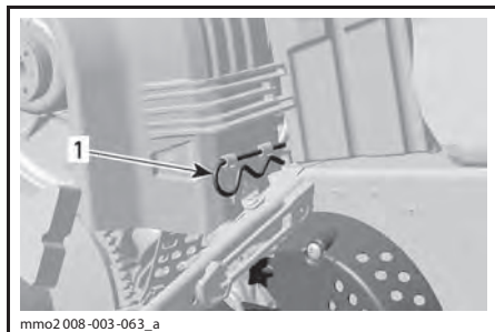
ТИПОВОЙ ВАРИАНТ 1. Проволоочный фиксатор
