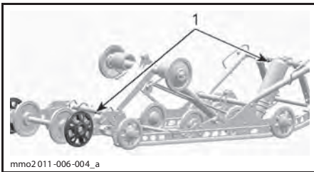
1. Пресс-маслёнки
