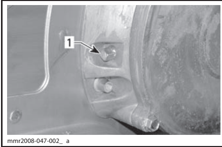
ТИПОВОЙ ВАРИАНТ — 600 HO E-TEC и 800R E-TEC 1. Магнитная пробка контрольного отверстия
