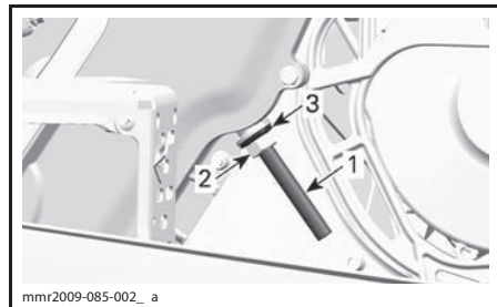
1. Регулировочный винт натяжения цепи 2. Контргайка 3. Уплотнительная шайба
