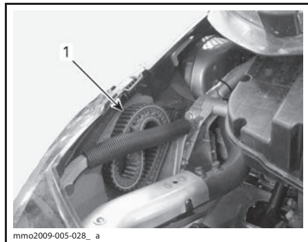
1. Правильно уложенный запасной ремень вариатора
