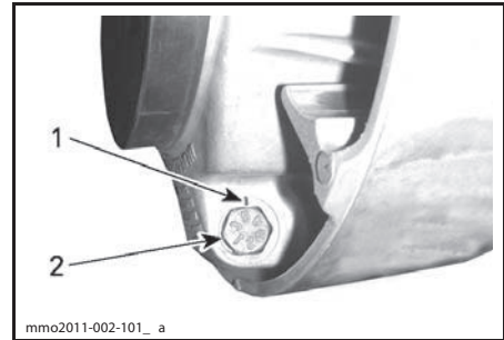
mmo2011-002-101_a НАСТРОЙКА ШКИВА
