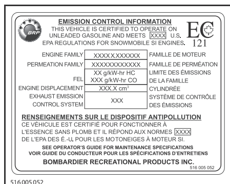
ТАБЛИЧКА СООТВЕТСТВИЯ 1 — В МОТОРНОМ ОТСЕКЕ
