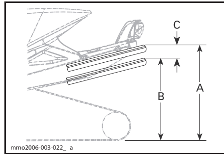
ТИПОВОЙ ВАРИАНТ — ПРАВИЛЬНАЯ РЕГУЛИРОВКА
