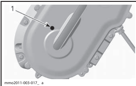
ТИПОВОЙ ВАРИАНТ — МОДЕЛИ 1200 4-TEC 1. Пробка контрольного отверстия
