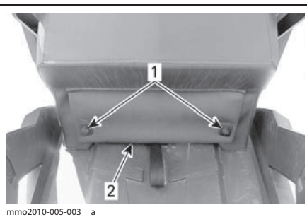
ЗАДНЯЯ ЧАСТЬ ПАССАЖИРСКОГО СИДЕНЬЯ 1. Фиксаторы 2. Крышка багажного отделения
