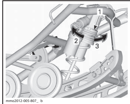
ТИПОВОЙ ВАРИАНТ — РЕГУЛЯТОР КОЛЬЦЕВОГО ТИПА
