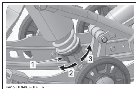
РЕГУЛЯТОР КУЛАЧКОВОГО ТИПА — АМОТИЗАТОР MOTION CONTROL
