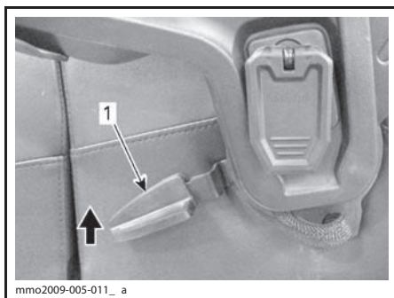
1. Блокировочный рычаг спинки
