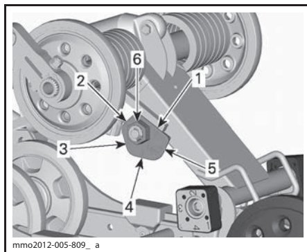
ПОДВЕСКА rMOTION БЕЗ ВЫНОСНЫХ РЕГУЛИРОВОЧНЫХ ЭЛЕМЕНТОВ — ЛЕВАЯ СТОРОНА
