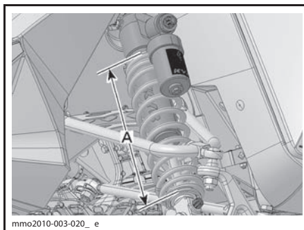
1. Максимум 270 мм, лыжи подняты над землёй
