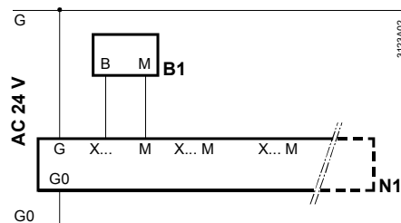
Схема 1: Измерительная часть с пассивным датчиком
