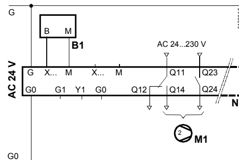
Схема 5: Подключение 2-скоростного вентилятора
