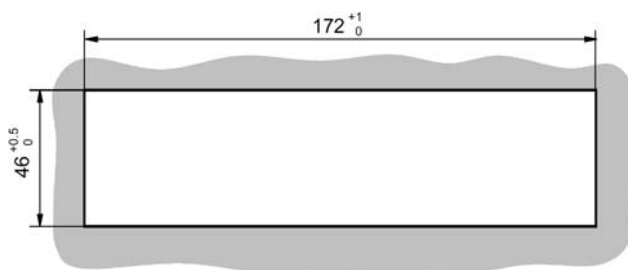
Разметка отверстия в панели управления для внешнего управления
