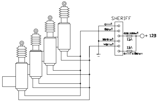
СХЕМА УПРАВЛЕНИЯ ЭЛЕКТРОПРИВОДАМИ ЗАМКОВ ДВЕРЕЙ ПРИ ПОШАГОВОМ (РАЗДЕЛЬНОМ) ОТПИРАНИИ ВОДИТЕЛЬСКОЙ И ПАССАЖИРСКИХ ДВЕРЕЙ АВТОМОБИЛЯ.
