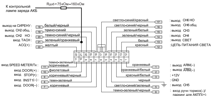
СХЕМА СОЕДИНЕНИЙ В РЕЖИМЕ АВТОЗАПУСКА БЕЗ ИСПОЛЬЗОВАНИЯ ДОПОЛНИТЕЛЬНОЙ ЦЕПИ IGN OUT
