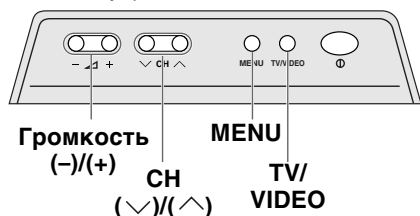
Панель управления основного блока
