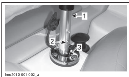
1. Опора кормового фонаря 2. Винтовая головка опоры 3. Шпоночная канавка
