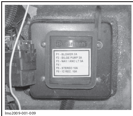
ПЕРЕДНИЙ БЛОК ПРЕДОХРАНИТЕЛЕЙ
