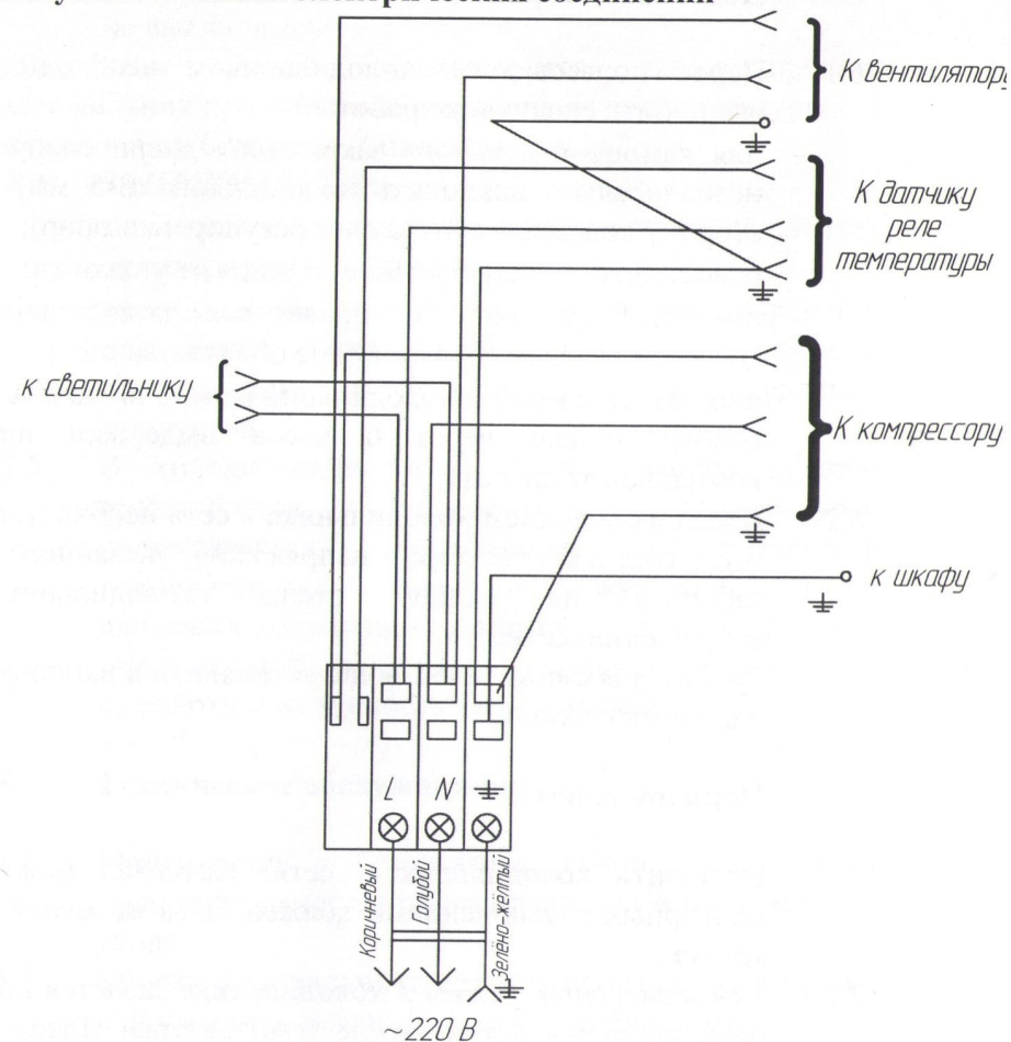
Рисунок 2 – Схема электрических соединений
