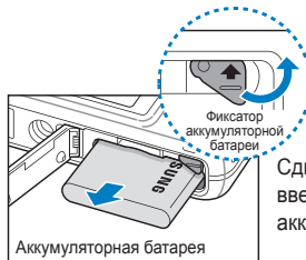
Аккумуляторная батарея
