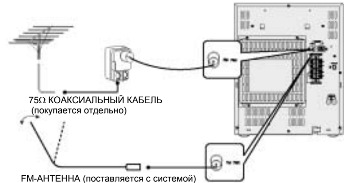
FM-АНТЕННА (поставляется с системой)
