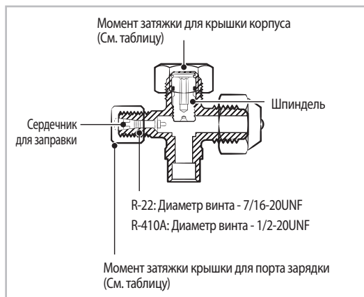
Устройство для испытания для наружного блока
