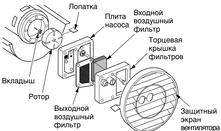
Рис. 24. Расположение ротора, нагреватели мощностью 30 и 44 кВт
