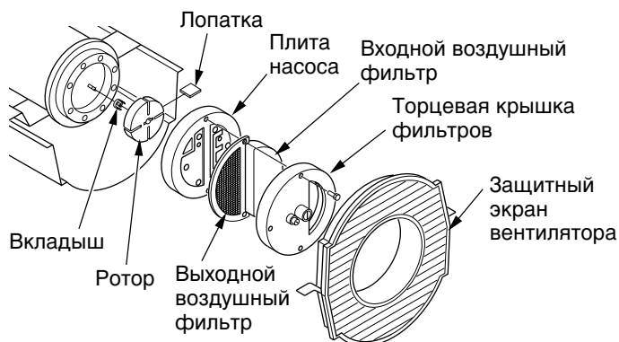
Рис. 23. Расположение ротора, нагреватели мощностью 10 и 20 кВт
