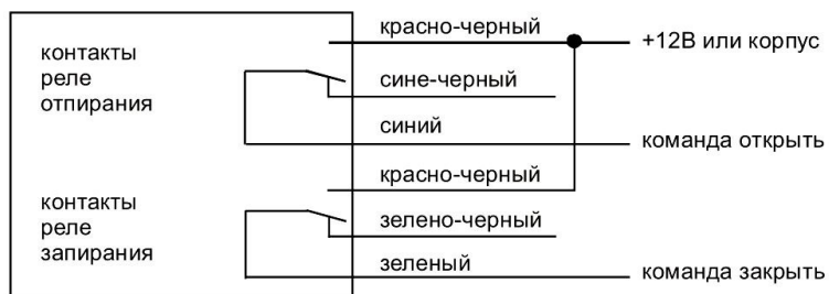
Схема подключения к системе запираения с положительным или отрицательным управлением
