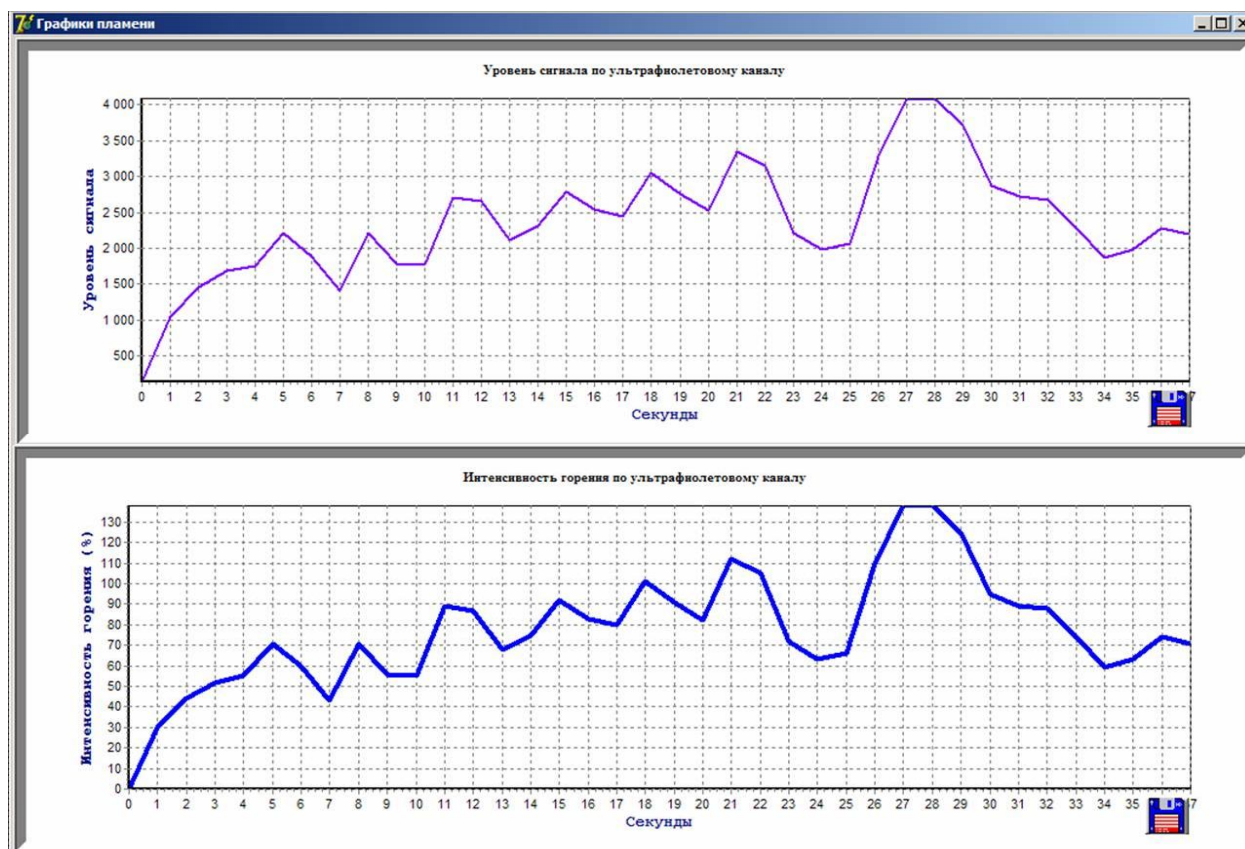
Рис.2 Графики пламени.
