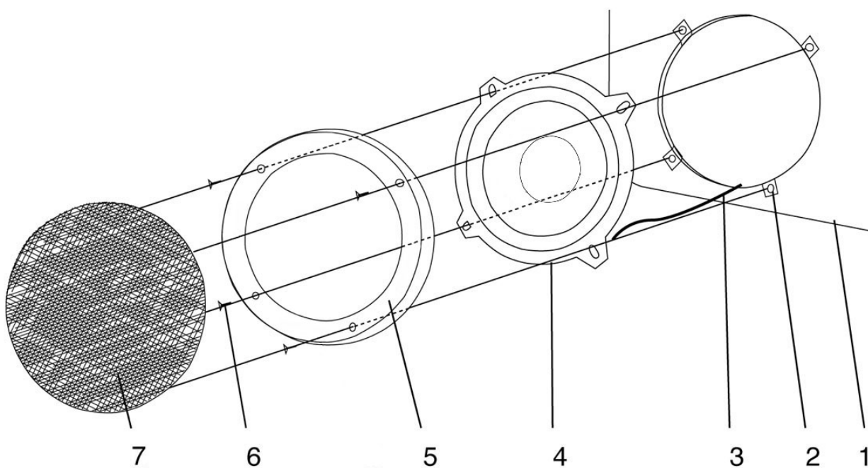
Рис.2. Схема установки НЧ-динамика.
