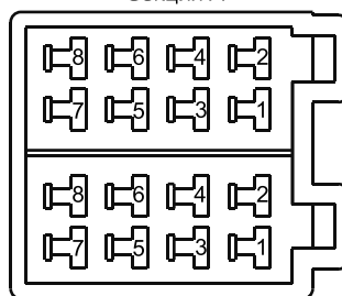
Расположение контактов разъема ISO:
