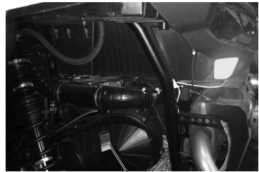
Загрязнение вариатора
